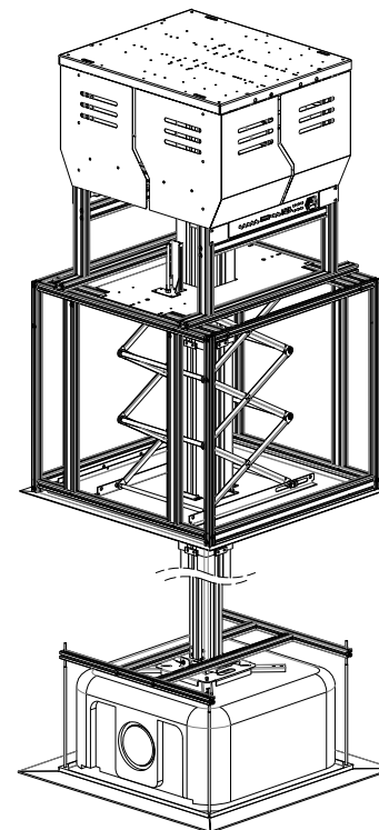
伸长图
